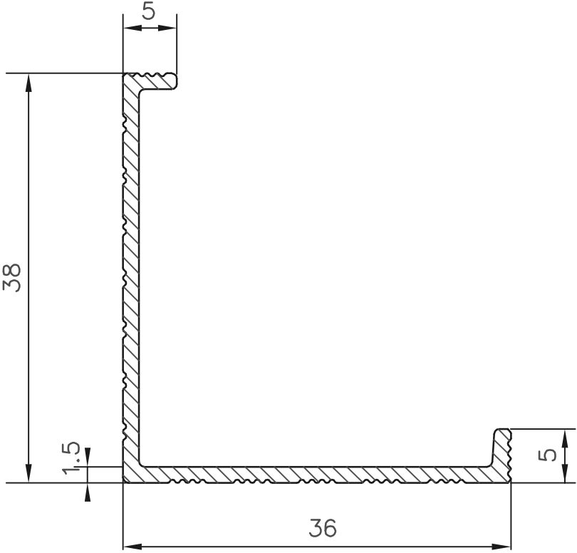
Abstellwinkel 38/36/1,5 mm M = 2:1
