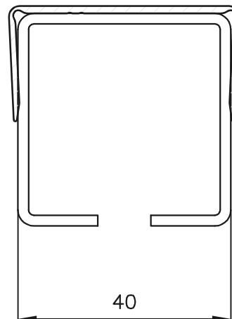
Aufsatzprofil auf Schaltwartenprofil aufgesetzt M = 1:1
