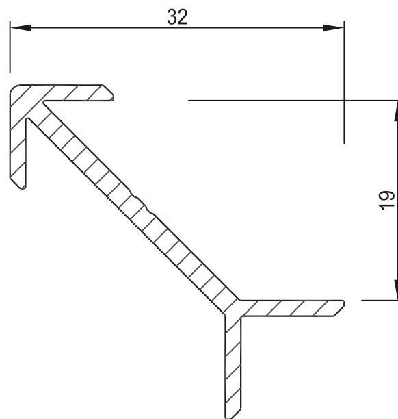
Eckausgleichsprofil
