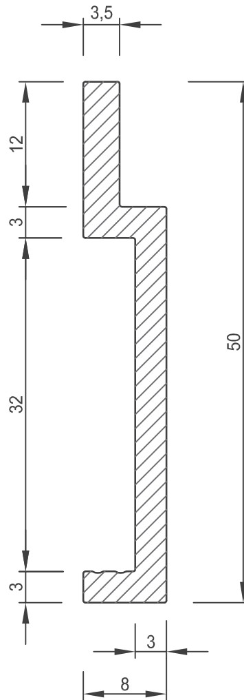
Einhängeprofil M = 2:1
