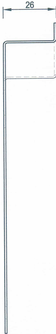
Seitenansicht M = 1:1
