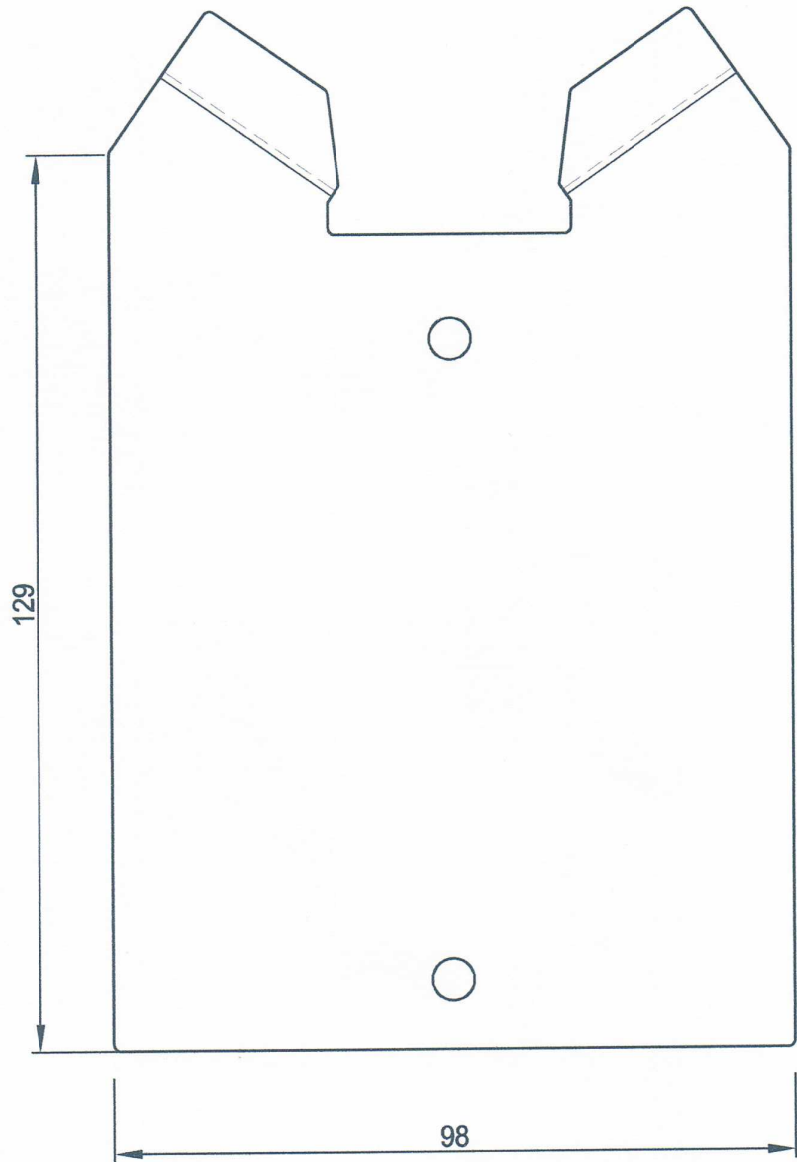
Vorderansicht M = 1:1
