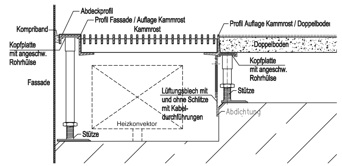
Querschnitt Konvektorgraben M = 1:5
