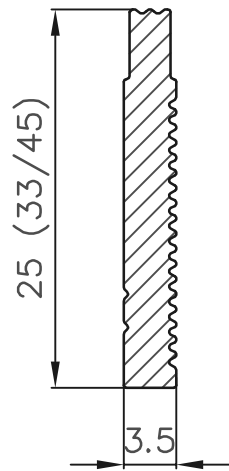
Kombi-Belagtrennleiste M = 2:1
